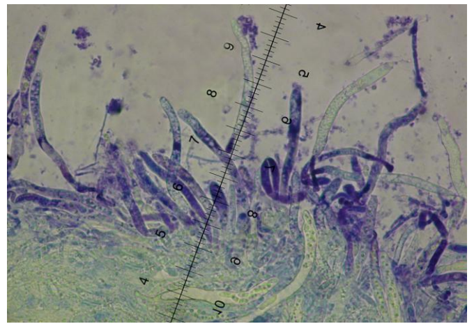
Bleu de crésyl
